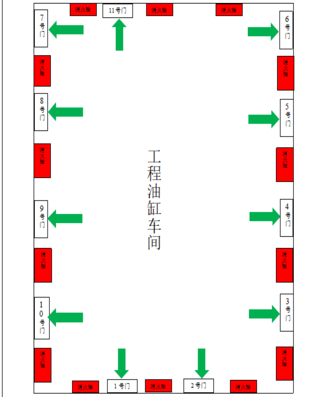
工程油缸车间应急逃生及消防器材布设图
